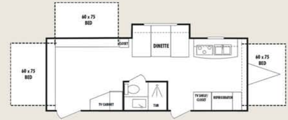
23CR •UVW 4570 • Length 26'3"
