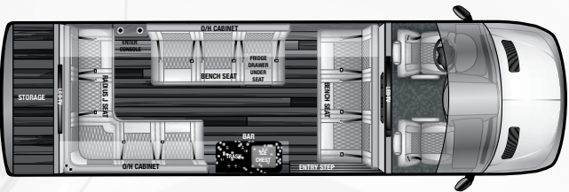
12LI/12LIA
